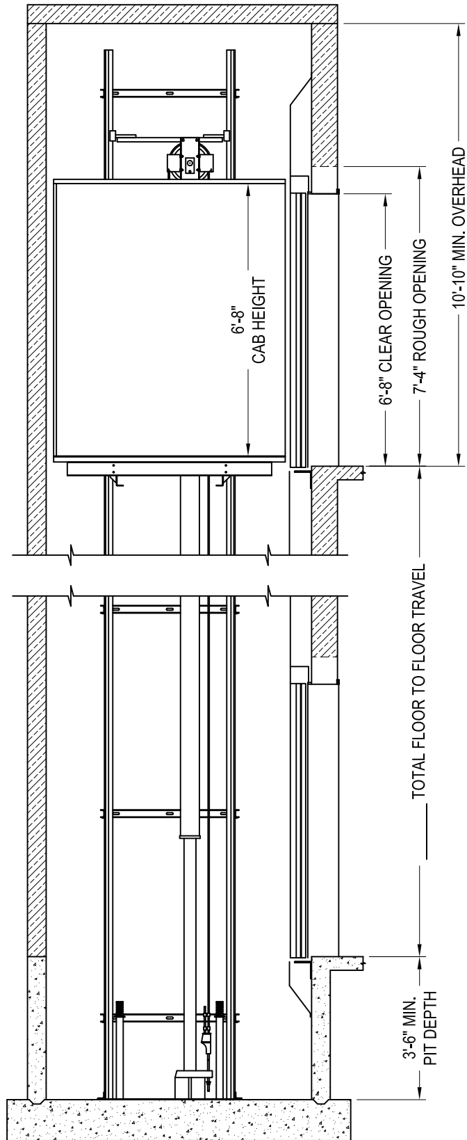
SECTION A-A
