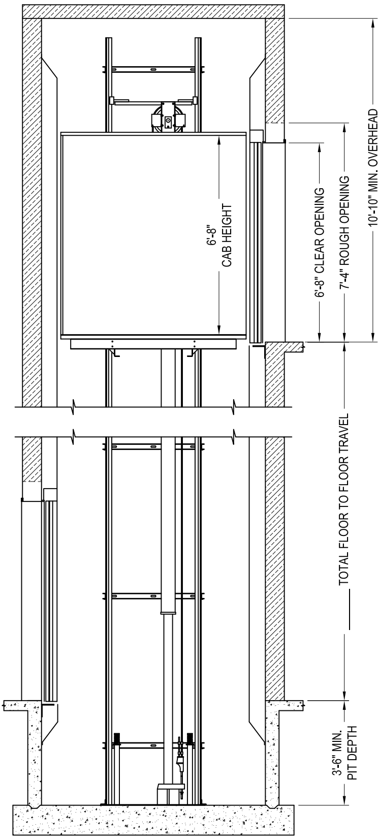
SECTION A-A
