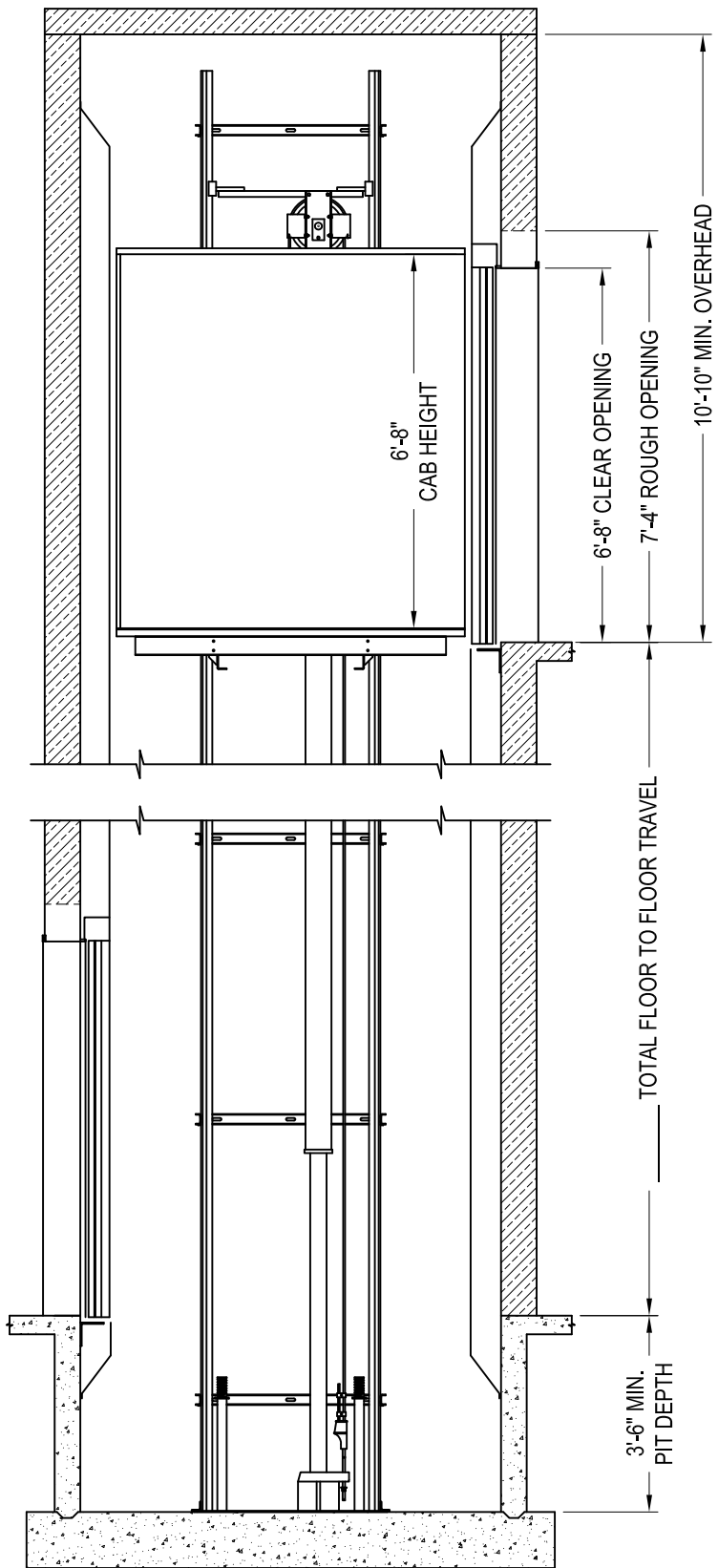
SECTION A-A
