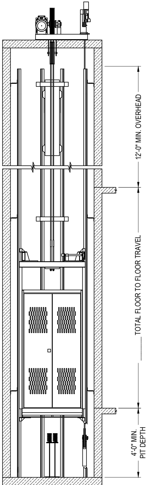
SECTION A-A
