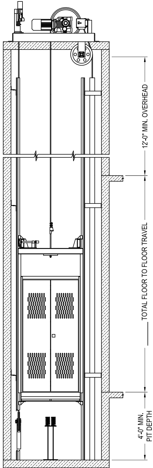
SECTION A-A
